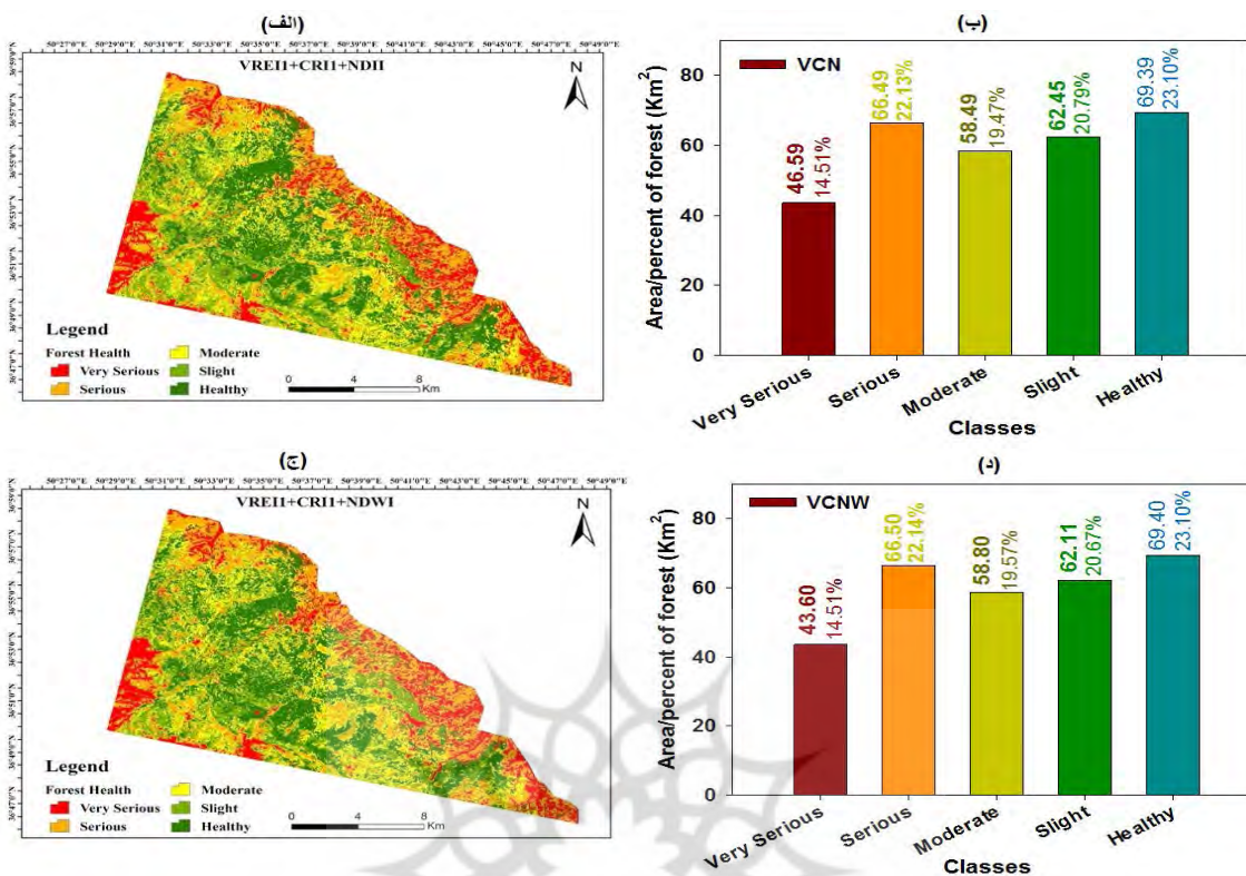
نگاره ۱۲: مناطق ریسک‌پذیر جنگلی، الف و ب) ترکیب شاخص‌های VCN، ج و د) ترکیب شاخص‌های VCNW
