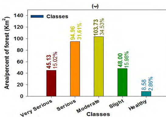
نگاره ۴: مناطق ریسک‌پذیر جنگلی حاصل از استخراج شاخص منفرد TVI
