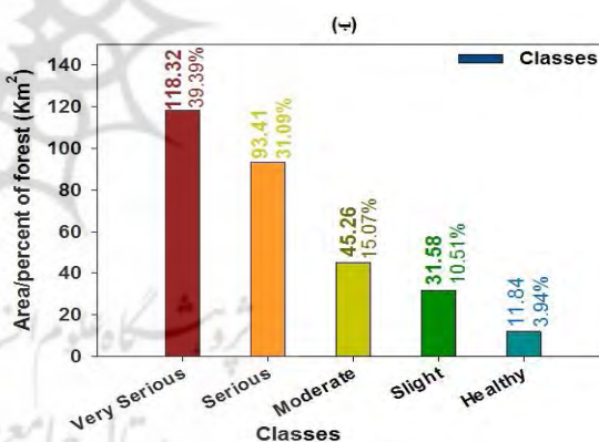
نگاره ۳: مناطق ریسک‌پذیر جنگلی حاصل از استخراج شاخص منفرد VREII
