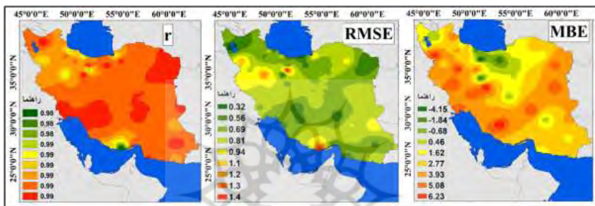
شکل (۲). کارایی مدل MPI-ESM-LR براساس درستی سنجی آماری داده‌های دمای مدل و داده‌های ایستگاهی طی دوره آماری ۱۹۸۰-۲۰۰۵ با استفاده از سنجه‌های آماری
