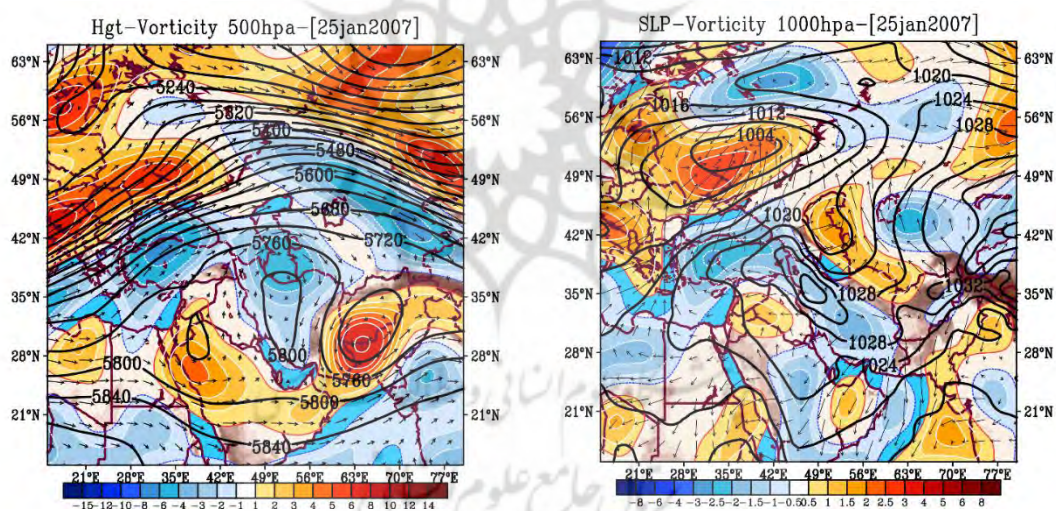
شکل ۴- وضعیت فشار تراز دریا و تاوایی سطح ۱۰۰۰ هکتوپاسکال (سمت راست)، تاوایی و ارتفاع ژئوپتانسیل
