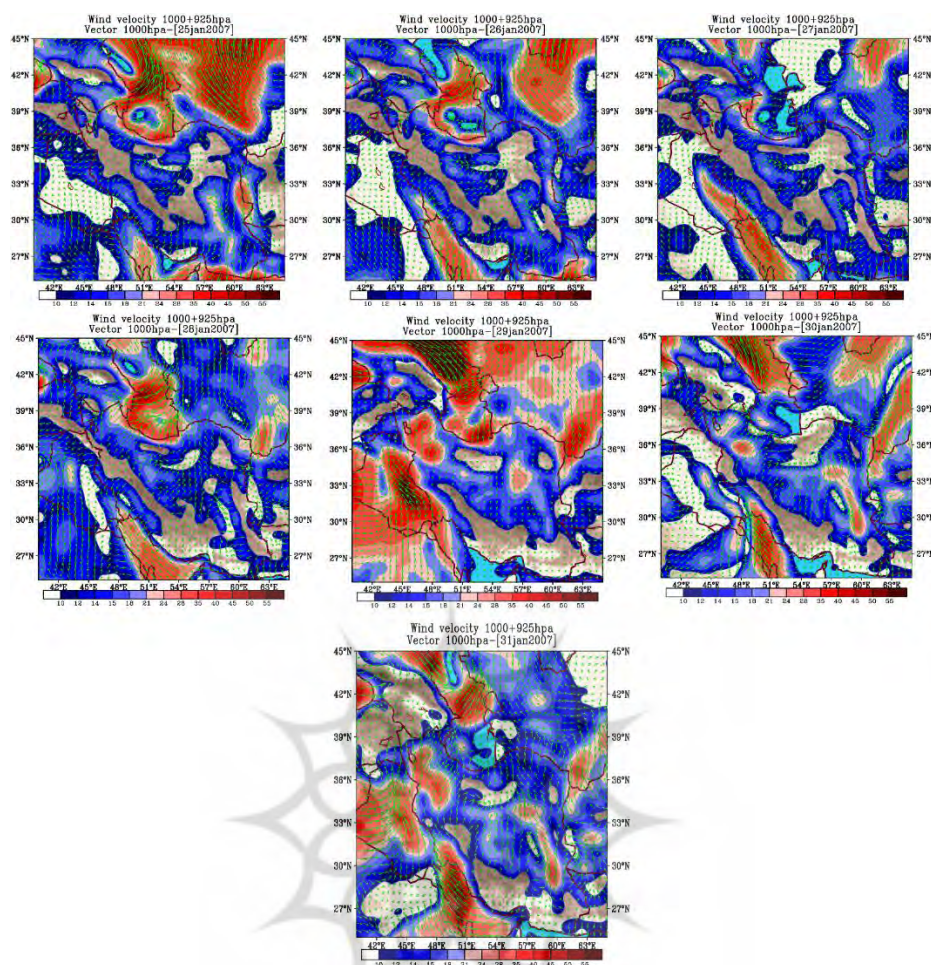
شکل ۱۱- وضعیت سرعت باد در لایه‌های زیرین جو (متوسط گیری شده برای تراز ۱۰۰۰ تا ۹۲۵ ه پ) از ۲۵ تا
