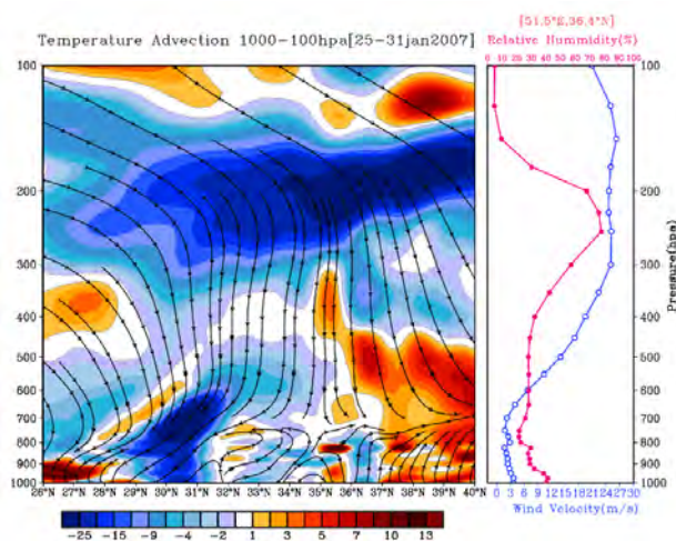
شکل ۱۴- نمودار مقطع قائم فرارفت دما برای طول ۵۱.۵ درجه شرقی و عرض ۲۶ تا ۴۰ درجه شمالی (سمت چپ)، نمودار مقطع قائم تغییرات رطوبت و سرعت باد برای نقطه ۵۱.۵ درجه شرقی و ۳۶.۴ درجه شمالی (سمت راست)-متوسط گیری شده برای کل دوره
