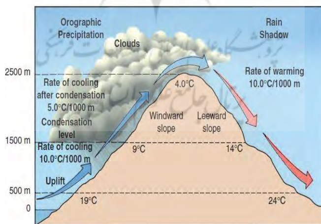
شکل ۱- اثر توپوگرافی بر روی توده‌ها در برخورد با کوهستان
