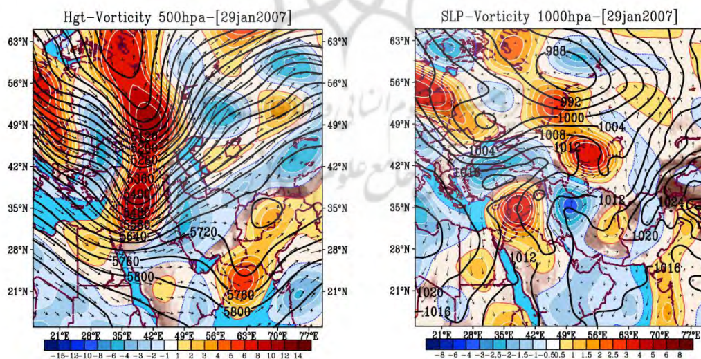
شکل ۸- وضعیت فشار تراز دریا و تاوایی سطح ۱۰۰۰ هکتوپاسکال (سمت راست)، تاوایی و ارتفاع ژئوپتانسیل تراز ۵۰۰ هکتوپاسکال (سمت چپ) برای تاریخ ۲۹ ژانویه ۲۰۰۷
