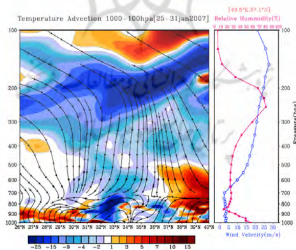
شکل ۱۳- نمودار مقطع قائم فرارفت دما برای طول ۴۹.۵ درجه شرقی و عرض ۲۶ تا ۴۰ درجه شمالی (سمت چپ)، نمودار مقطع قائم تغییرات رطوبت و سرعت باد برای نقطه ۴۹.۵ درجه شرقی و ۳۷.۱ درجه شمالی (سمت راست)-متوسط گیری شده برای کل دوره
