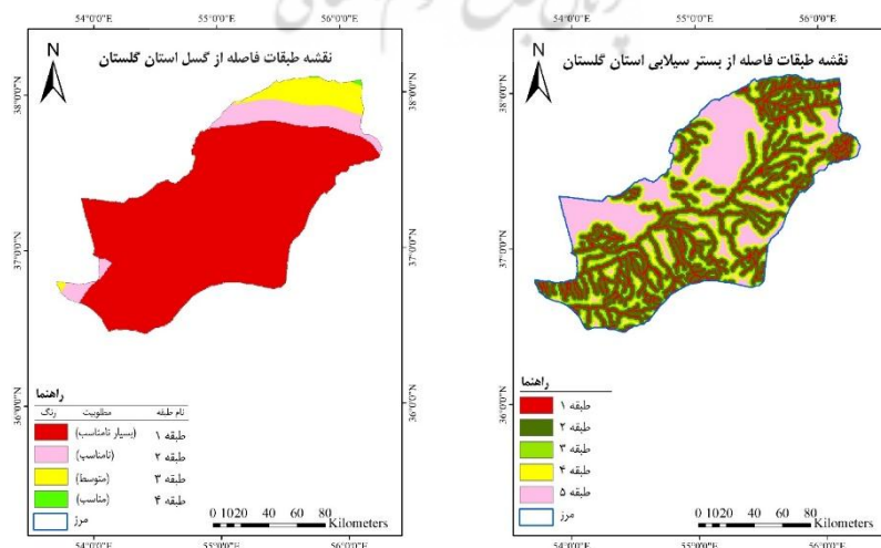
شکل ۱۰: الف) نقشه طبقه‌بندی فاصله از بستر سیلابی استان گلستان، ب) نقشه طبقه‌بندی فاصله از گسل استان گلستان
