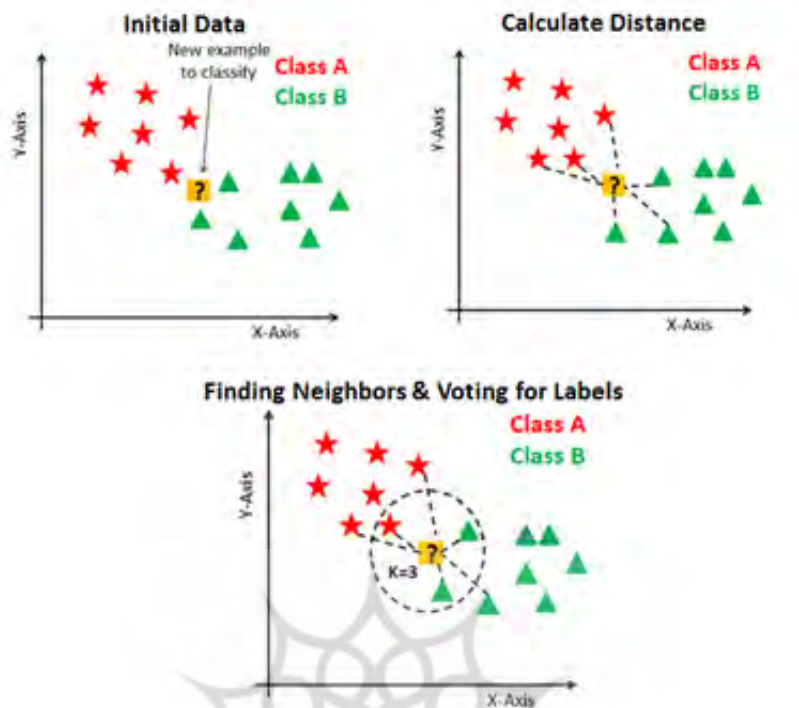
شکل ۱. الگوریتم k-نزدیک‌ترین همسایه
