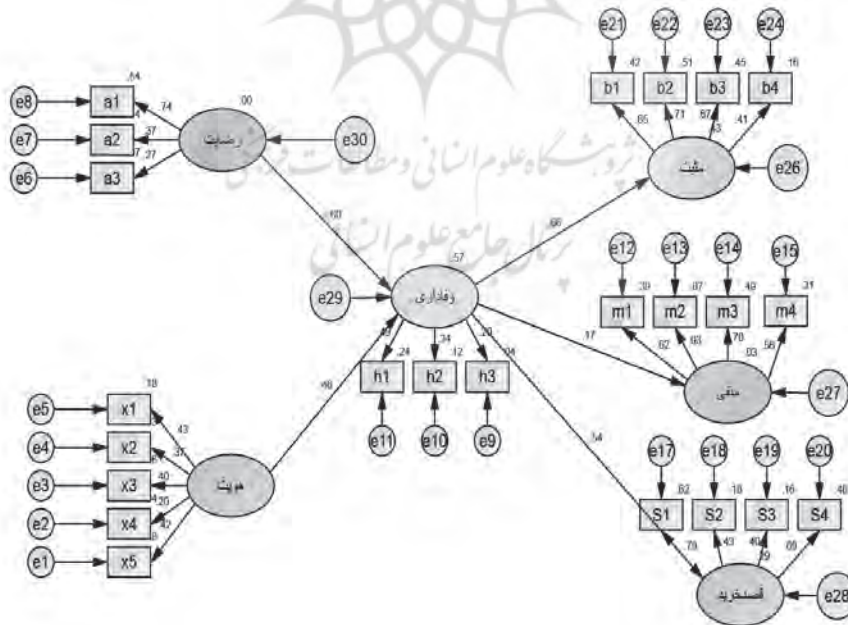
شکل ۱: مدل پژوهش
