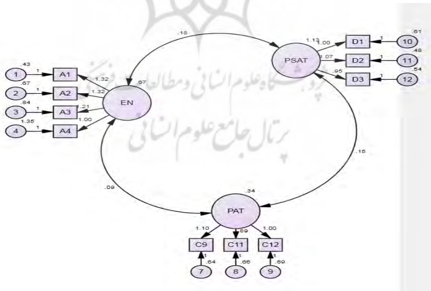
شکل ۲. مدل تحلیل عاملی تأییدی
