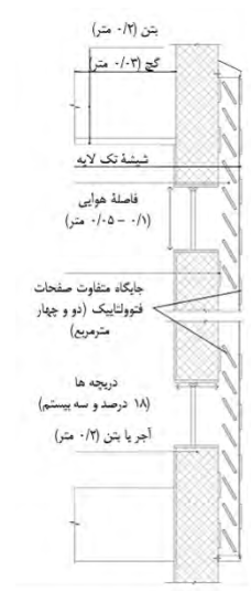
شکل ۵. مقطعی از دیوار ترومب فتوولتائیک
