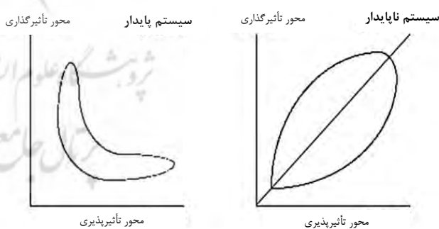
تصویر ۳. الگوی سیستم پایدار و ناپایدار. مأخذ: Godet, et al., 2003. به نقل از نعیمی و پورمحمدی، ۱۳۹۵.
