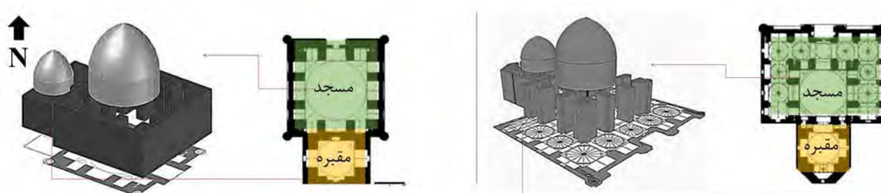
تصویر ۲. راست: پلان مسجد کبود شامل دو گنبد خانه در راستای محور شمالی-جنوبی؛ چپ: پلان مسجد حسن پادشاه شامل دو گنبدخانه در راستای محور شمالی-جنوبی. مأخذ: سربابی و همکاران، ۱۳۹۹.
