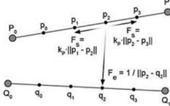
تصویر ۳. تقسیم خطوط مستقیم به چندین قسمت. نقاط به دست آمده همان اجزای تشکیل‌دهنده سیستم هستند. F_s : نیروی دافعه بین نقاط در هر خط، F_e : نیروی جاذبه بین نقاط متناظر در یک دسته خطوط، K_p : ضریبی است که میزان صلبیت خطوط را در تبدیل شدن به فنر کنترل می‌کند. مأخذ: Holten & Van Wijk, 2009.
