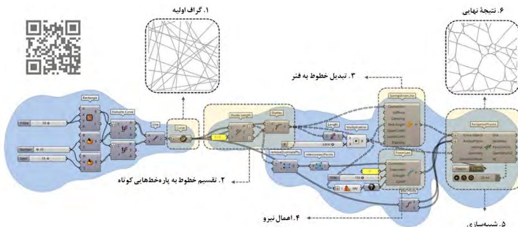
تصویر ۶. الگوریتم رشته‌های خیس در افزونه گرسپایر، به‌همراه بارکد نمایش شبیه‌سازی. مأخذ: نگارندگان.
