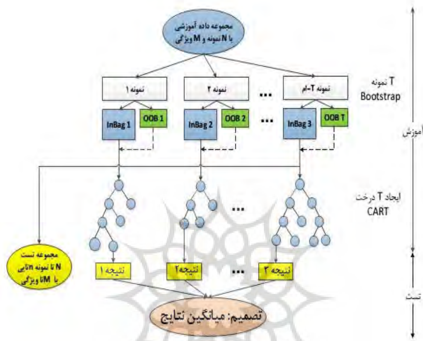
شکل ۳- ساختار الگوریتم جنگلی تصادفی. (Guo et al. 2011)
