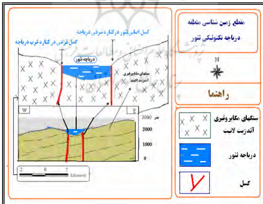
شکل (۳) در مقطع زمین شناسی حوضه دریاچه شکل گرفته در حالت گراهن
