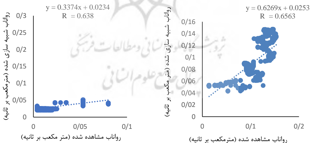
شکل (۸): همبستگی داده‌های رواناب مشاهده شده و شبیه‌سازی شده مدل در مرحله‌ی الف) واسنجی و ب) صحت‌سنجی در حوضه‌ی آبریز خنچه
