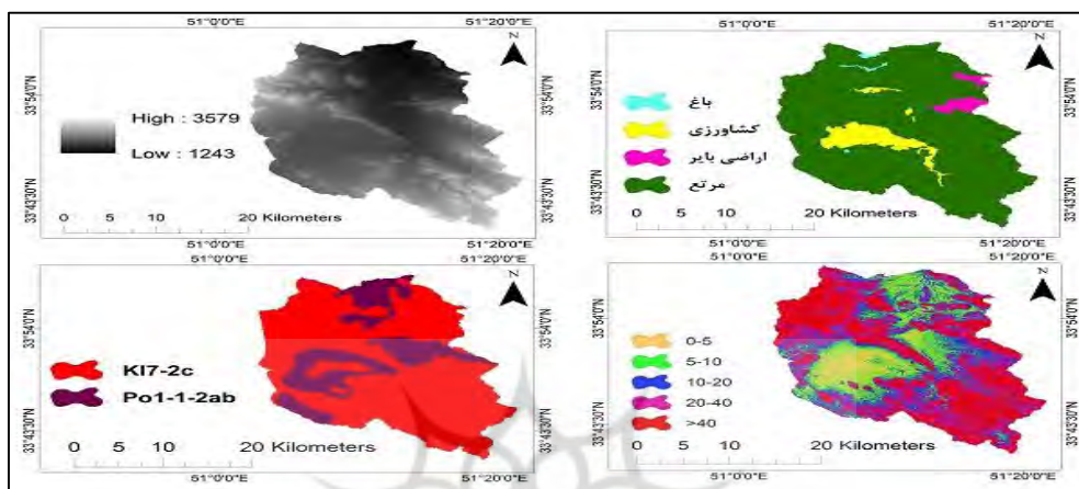
شکل (۲): نقشه‌های مکانی حوضه‌ی آبریز (خنچه)
