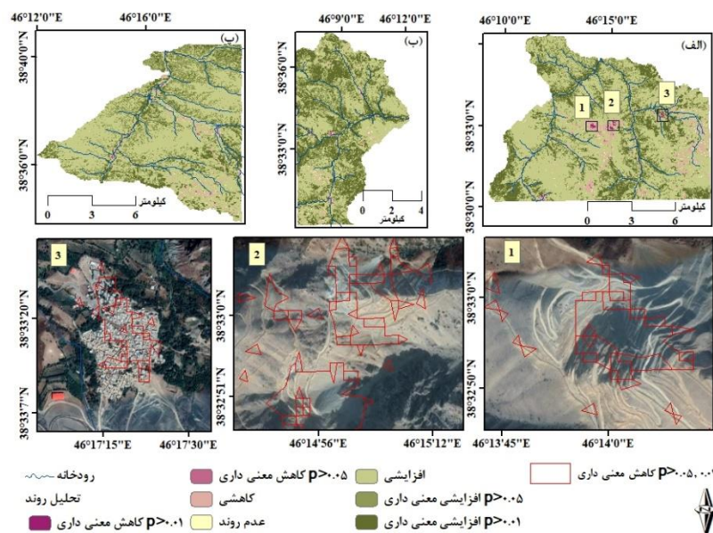
شکل (6): طبقه‌بندی روند در سطح اطمینان 95 و 99 درصد، (الف) منطقه 1، (ب) منطقه 2 و (ب) منطقه 3. شکل شماره 1-3 که از شکل الف منتج شده است نشان‌دهنده‌ی مناطق دارای روند کاهشی معنی‌داری پوشش گیاهی است. شکل 1 و 2 مناطق معدن‌کاوی شده و شکل 3 روستای اندریان است.
