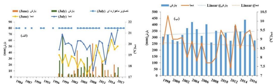
شکل (2): دما و بارش ماهانه در ایستگاه ورزقان و تاریخ تصاویر ماهواره‌ای استفاده شده (الف)، میانگین دمای سالانه و بارش سالانه (ب)
