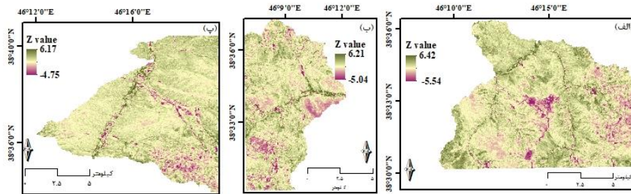
شکل (5): تغییرات روند پوشش گیاهی با استفاده از روش من-کندال، (الف) مقدار Z در منطقه 1، (ب) مقدار Z در منطقه 2 و (پ) مقدار Z در منطقه 3
