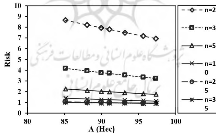
شکل (۳) نمودار ریسک در مقابل مساحت (منحنی فرمان) با عمر مفید مختلف
