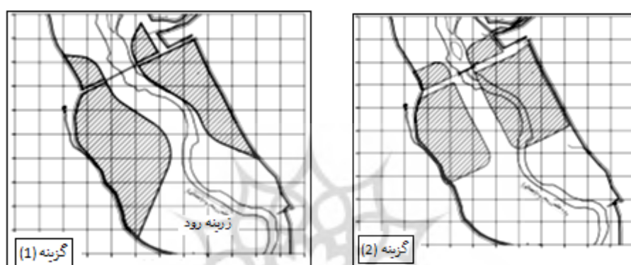
شکل (۴) نمایی از شرایط گزینه "یک" و "دو" بررسی طرح ساماندهی زربنه رود Fig(4) Scheme of the two alternatives in river training project of the Zarrinehrod
