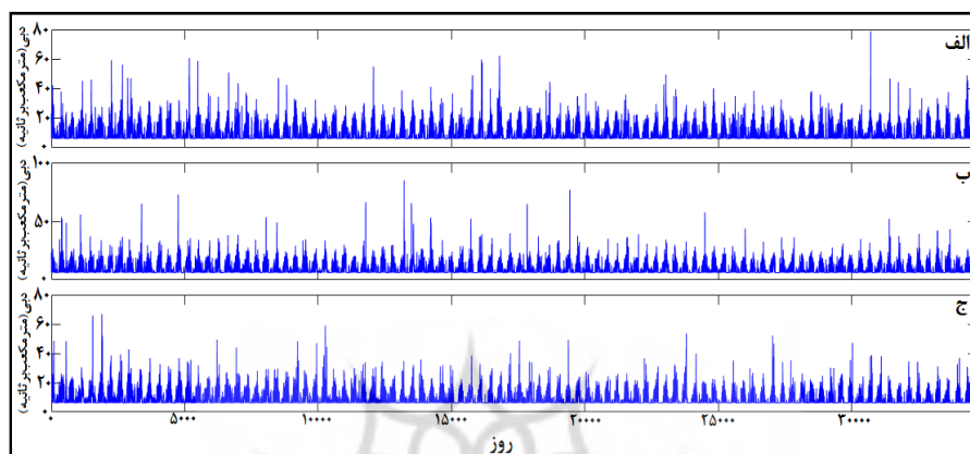
شکل (۹) نمودار مقادیر رواناب روزانه شبیه‌سازی شده برای سال ۲۱۰۰-۲۰۰۶ با به کارگیری سناریوهای الف: RCP 2.6 - ب: RCP 4.5 و ج: RCP 8.5
