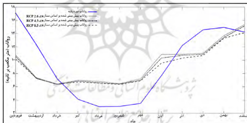
شکل (۱۱) نمودار مقادیر رواناب ماهانه شبیه‌سازی شده برای سال ۲۱۰۰-۲۰۰۶ با به کارگیری سناریوهای RCP 8.5 و RCP 4.5 – RCP 2.6
