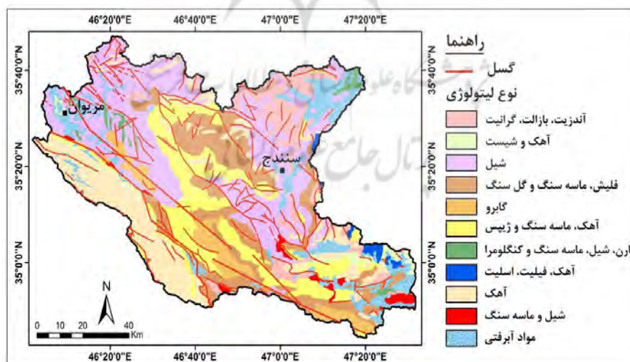
شکل (۲) نقشه‌ی زمین‌شناسی حوضه‌ی رودخانه سیروان
