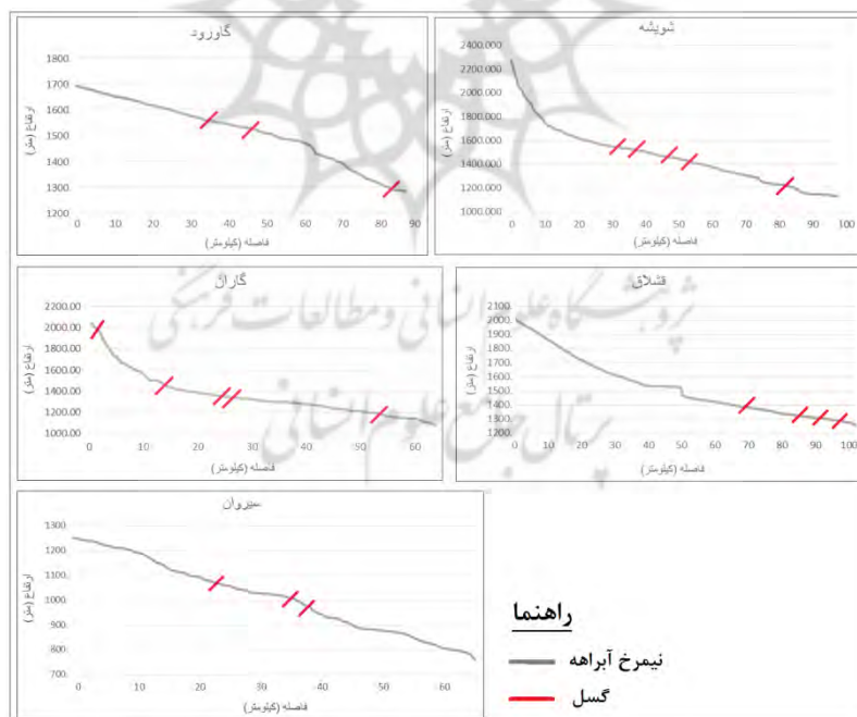
شکل (۵) نیمرخ طولی رودخانه‌های اصلی زیرحوضه‌های رودخانه سیروان
