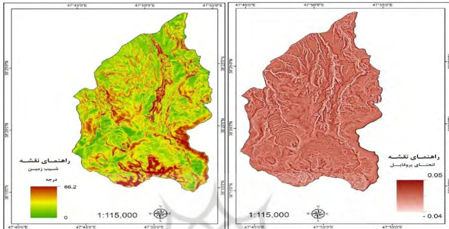
شکل (۲) لایه شیب زمین
