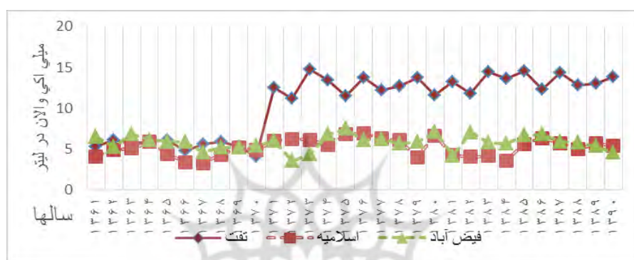
شکل (۶) روند تغییرات مجموع کاتیون‌ها (MEq) در ایستگاه‌های تفت، اسلامیة و فیض‌آباد
