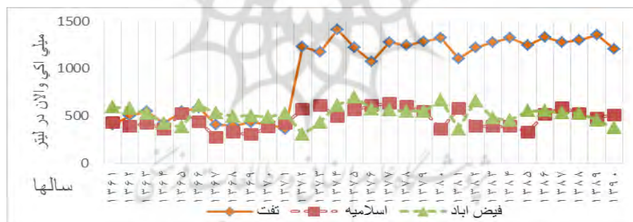
شکل (۷) روند تغییرات هدایت الکتریکی (MEq) در ایستگاه‌های تفت، اسلامیة و فیض‌آباد
