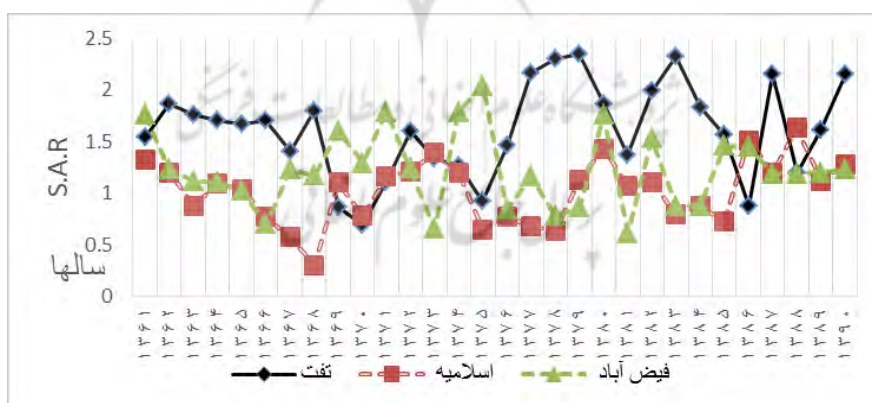
شکل (۹) روند تغییرات میزان SAR در ایستگاه‌های تفت، اسلامیه و فیض‌آباد
