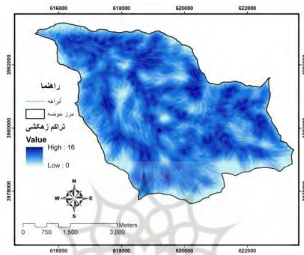
شکل (۲) نقشه‌ی تراکم زهکشی حوضه‌ی بهرستاق
