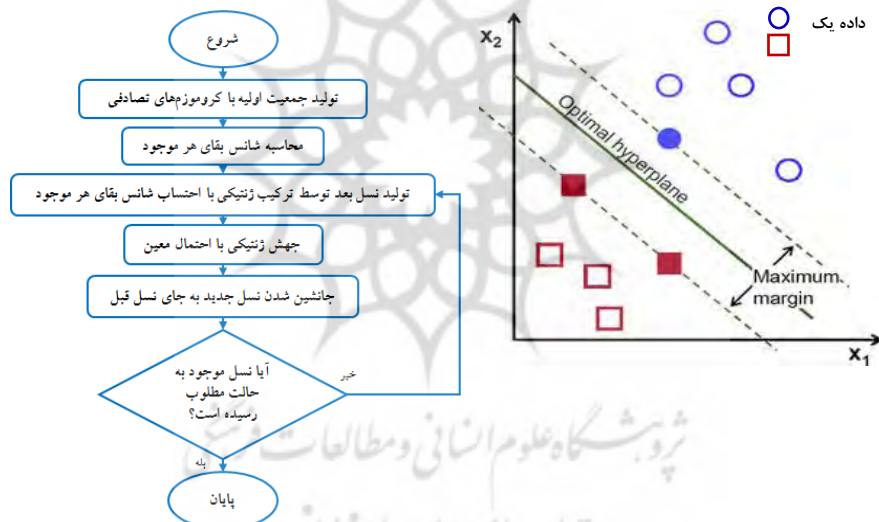
شکل (۱) حل معادله با رگرسیون SVR شکل (۲) فلوچارت الگوریتم ژنتیک
