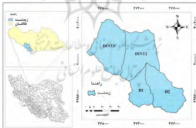
شکل (۱) موقعیت حوضه آبخیز زیدشت در کشور، استان و منطقه
