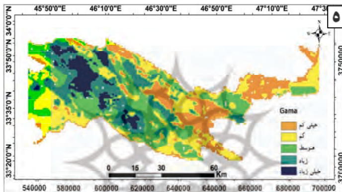
شکل (۱۰) نقشه‌های پهنه‌بندی نهایی آب زیرزمینی با روش منطق فازی (ه) عملگر Gama.
