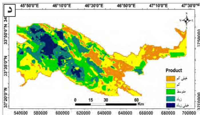
شکل (۹) نقشه‌های پهنه‌بندی نهایی آب زیرزمینی با روش منطق فازی (جد) عملگر Product
