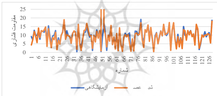
شکل ۵- مقایسه مقادیر آزمایشگاهی و پیش‌بینی شده توسط شبکه عصبی ساخته شده. Figure 5- Comparison of experimental and predicted values by the constructed neural network.
