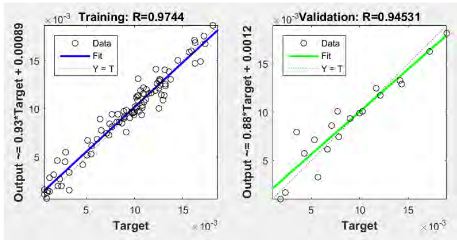
شکل ۴-مقایسه مقادیر حقیقی مقاومت فشاری بتن با مدل ساخته شده برای داده‌های آموزش و اعتبار سنجی. Figure 4-Comparison of the actual values of concrete compressive strength with the built model for training and validation data.
