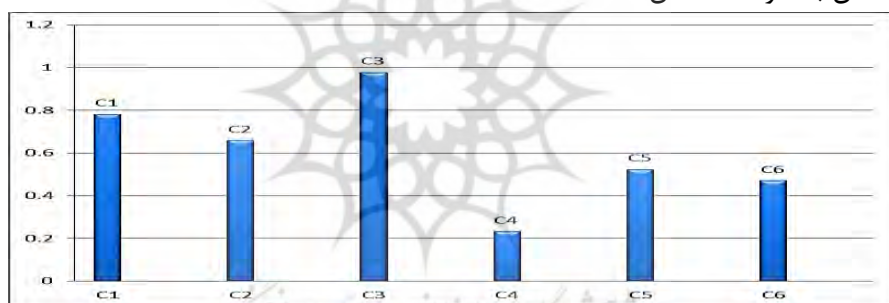
نمودار (۲) رتبه‌بندی ترتیب مطلوبیت
