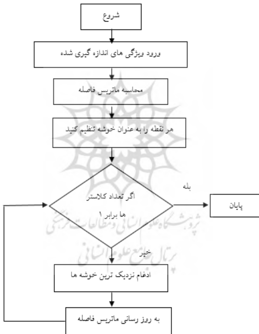
شکل ۳: فلوجارت الگوریتم AGNES
