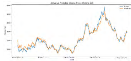
CNN
