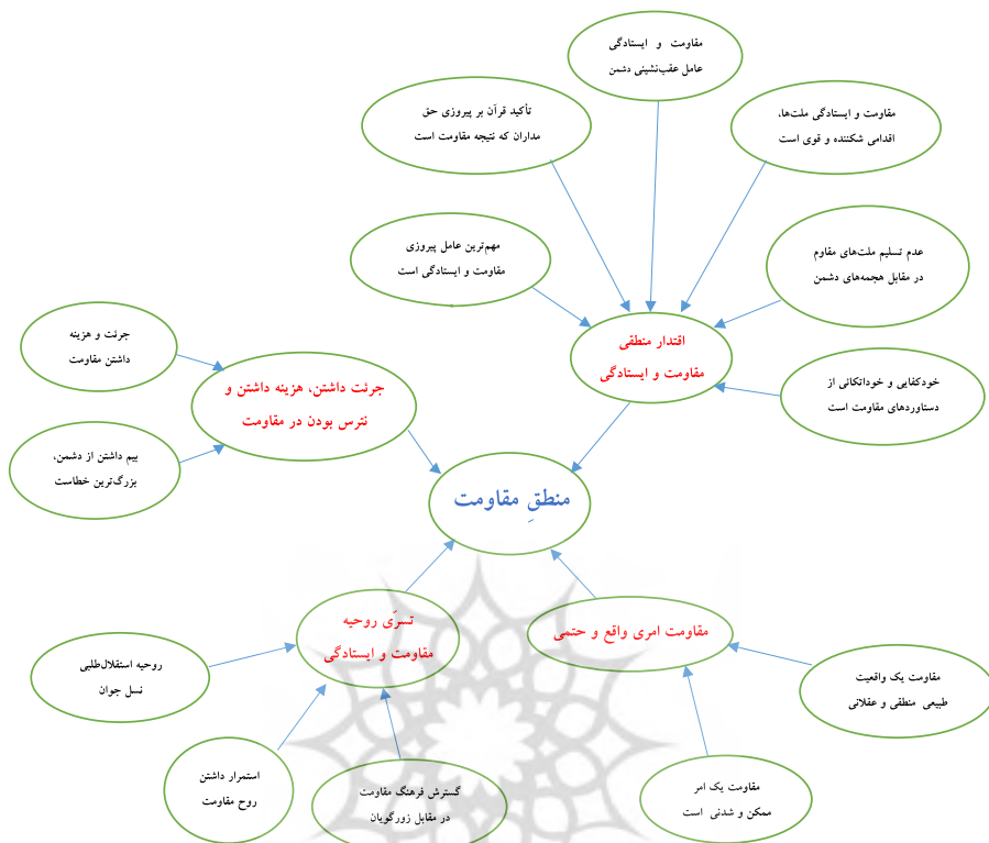
شکل ۱- شبکه مضامین «منطق مقاومت» در دیدگاه مقام معظم رهبری
