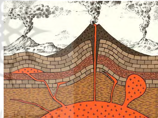
الشكل ٢ - رسم توضيحي بسيط لتكوين الجبال النارية وارتفاع سطح الأرض بأعمدة من مادة منصهرة متصلة في العمق ومتصلة في الأرض.
