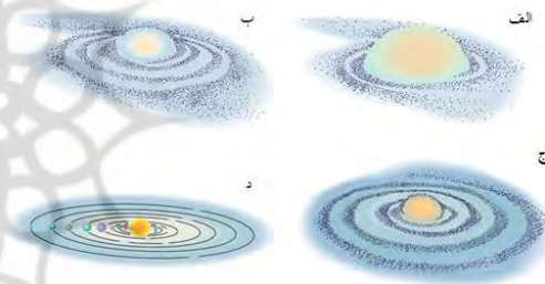
الشكل ١ - مراحل تكوين وتطور الشمس وكواكب المجموعة الشمسية الأخرى
