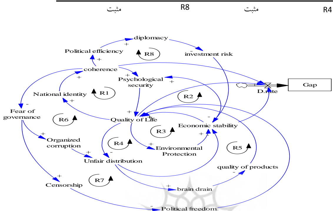
شکل (۴) مدل در حالت مرجع
