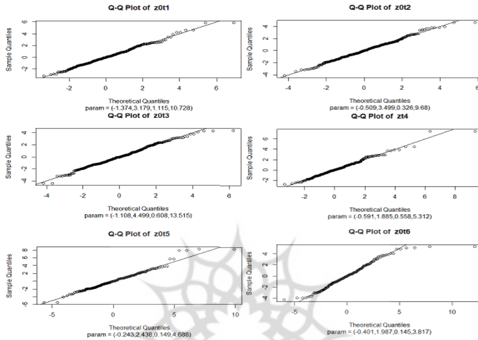
شکل ۳- نمودار چندک-چندک سری‌های بازدهی شاخص‌های صنایع فیلتر شده ( z_t ) در مقابل توزیع جنرال
