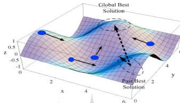
شکل ۲- نمایشی از بهترین راحل بهینه‌یابی محلی و سراسری
