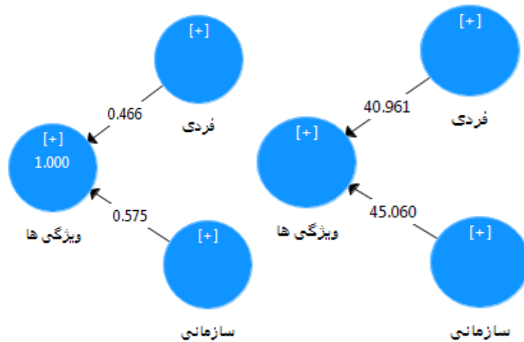
شکل ۳. حالت معناداری (چپ) و استاندارد (راست) مدل اندازه‌گیری ضربه روحی (Source: By author)
