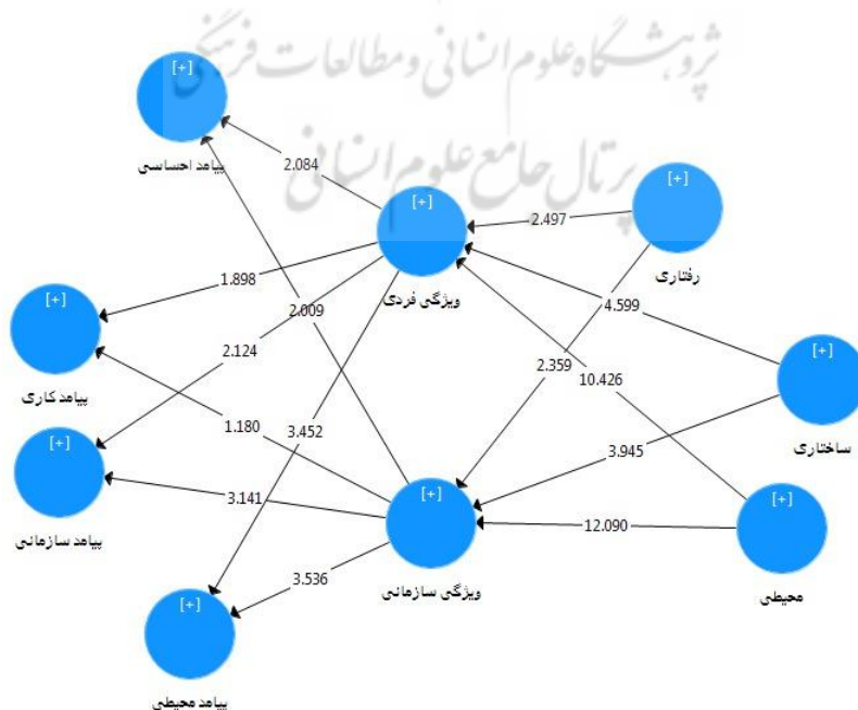
شکل ۶. حالت معناداری مدل ساختاری در حالت جزئی (Source: By author)
