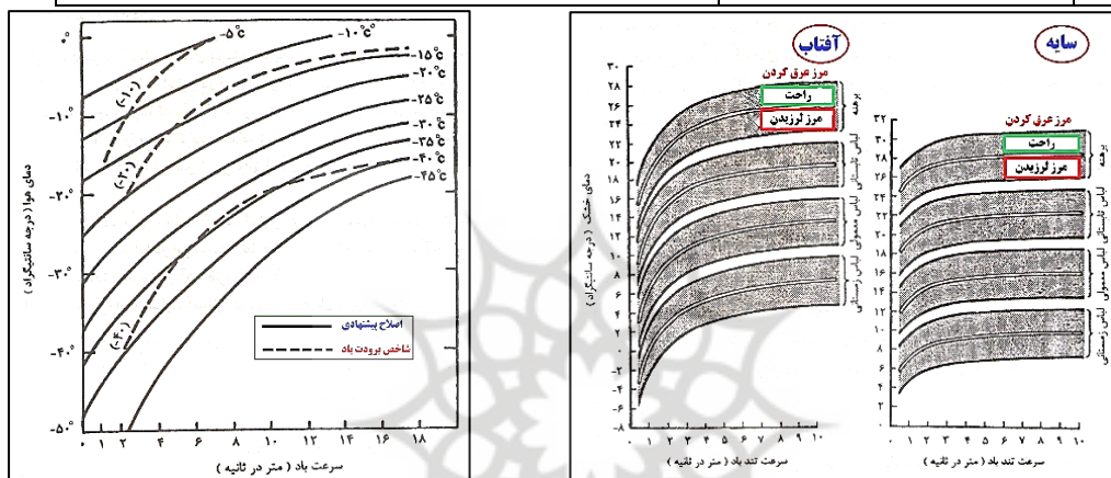
شکل (۱): معیار آسایش پن واردن در سایه و آفتاب
