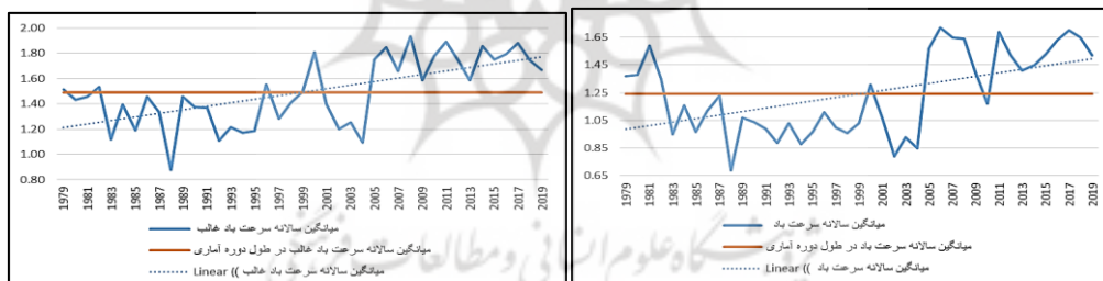
شکل (۵): تغییرات سالانه سرعت باد در شهر رشت
