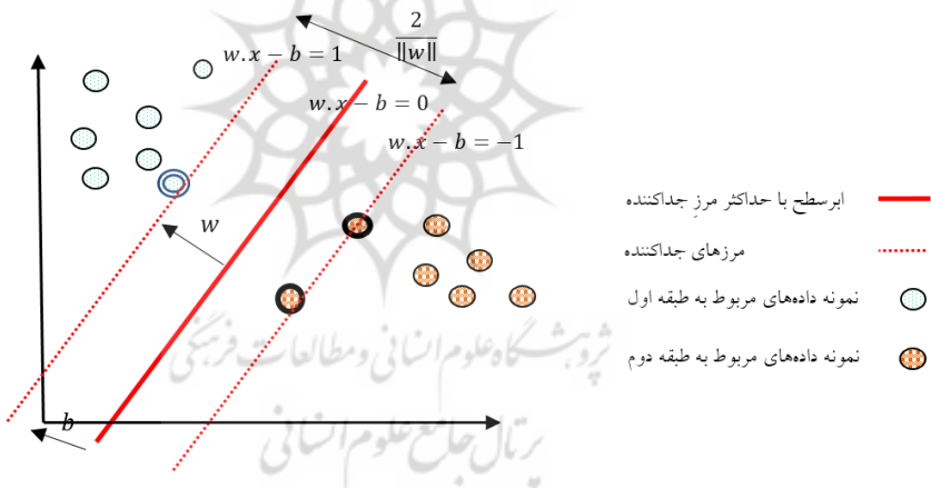
شکل ۲- ابرسطح با حداکثر مرز جداکننده به همراه مرزهای جداکننده برای طبقه‌بندی
