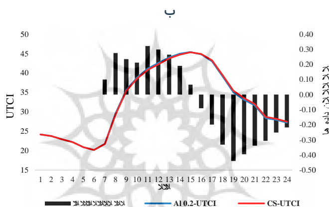
شکل (۶): مقایسه شاخص‌های آسایش حرارتی بین حالت Al 0.8 با CS (الف) شکل مربوط به شاخص PET و (ب) شاخص UTCI
