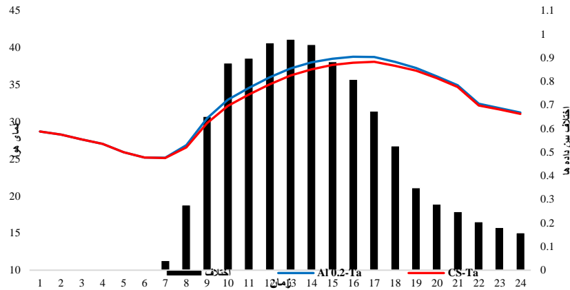
شکل (۴): مقایسه داده‌های بین دو حالت وضع موجود و آلبدو ۰٫۲ و اختلاف بین داده‌های (الف) داده‌های دمای هوا و (ب) رطوبت نسبی
