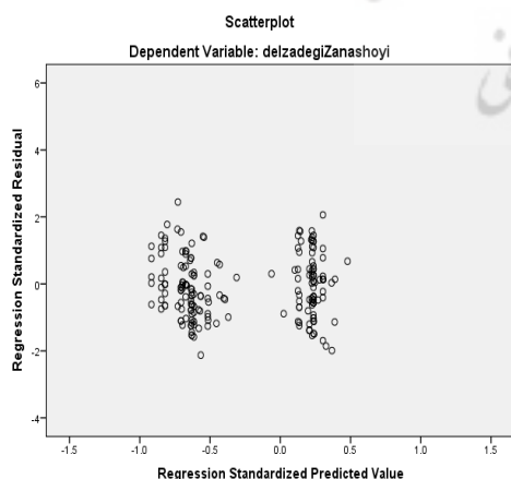
شکل ۴-۲ نمودار پراکنندگی باقیمانده‌های استاندارد
