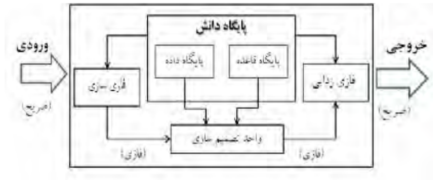
شکل ۱: اجزای سیستم استدلال فازی
