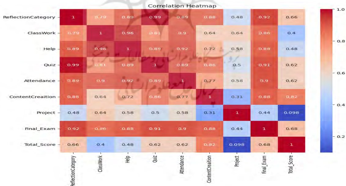
شکل ۷: وابستگی ویژگی‌های مختلف به یک دیگر (داده‌های کامپیوتر)
