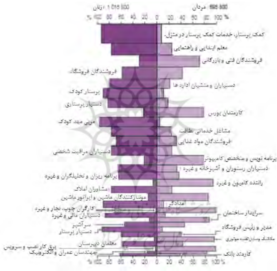
نمودار ۱. تقسیم کار جنسیتی زنان و مردان در سوئد
