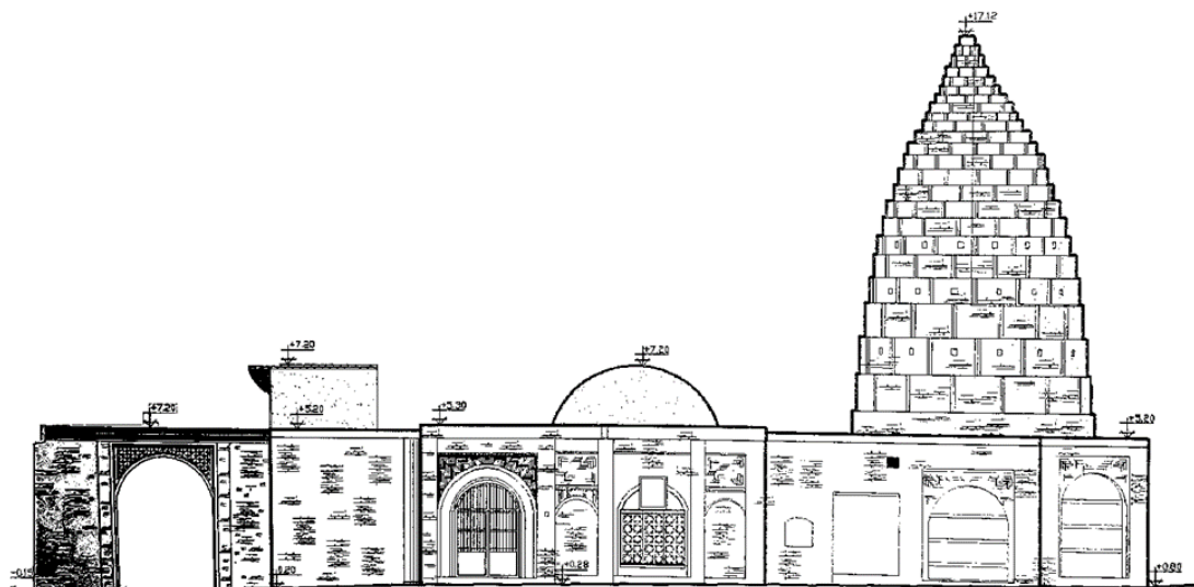
شکل ۳. طرح نمای شمالی امامزاده (Source: Lorestan Cultural Heritage Archive)
