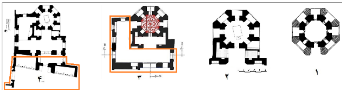
شکل ۱۱. پلان ۱. پلان فرضی اولیه بنا و مراحل توسعه آن (دوره سلجوقی) پلان ۲. الحاق ورودی به گنبدخانه پلان ۳. الحاق شبستان عرضی و فضای غربی پلان ۴. ایجاد ایوان و زائرسرا و درگاه ورودی (مأخذ: آرشیو میراث فرهنگی لرستان، تغییرات از نگارنده).
