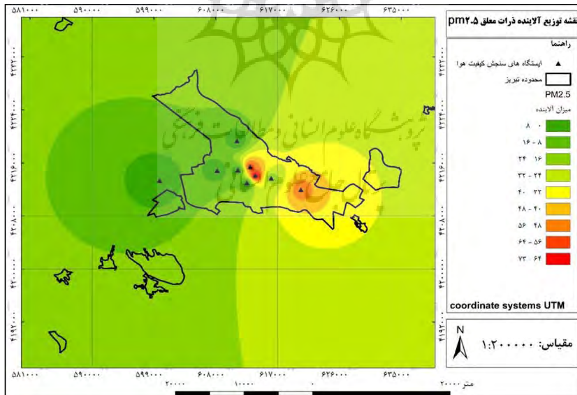
شکل ۷ نقشه توزیع آلاینده ذرات معلق PM2.5 در تبریز، مأخذ: نگارندگان
