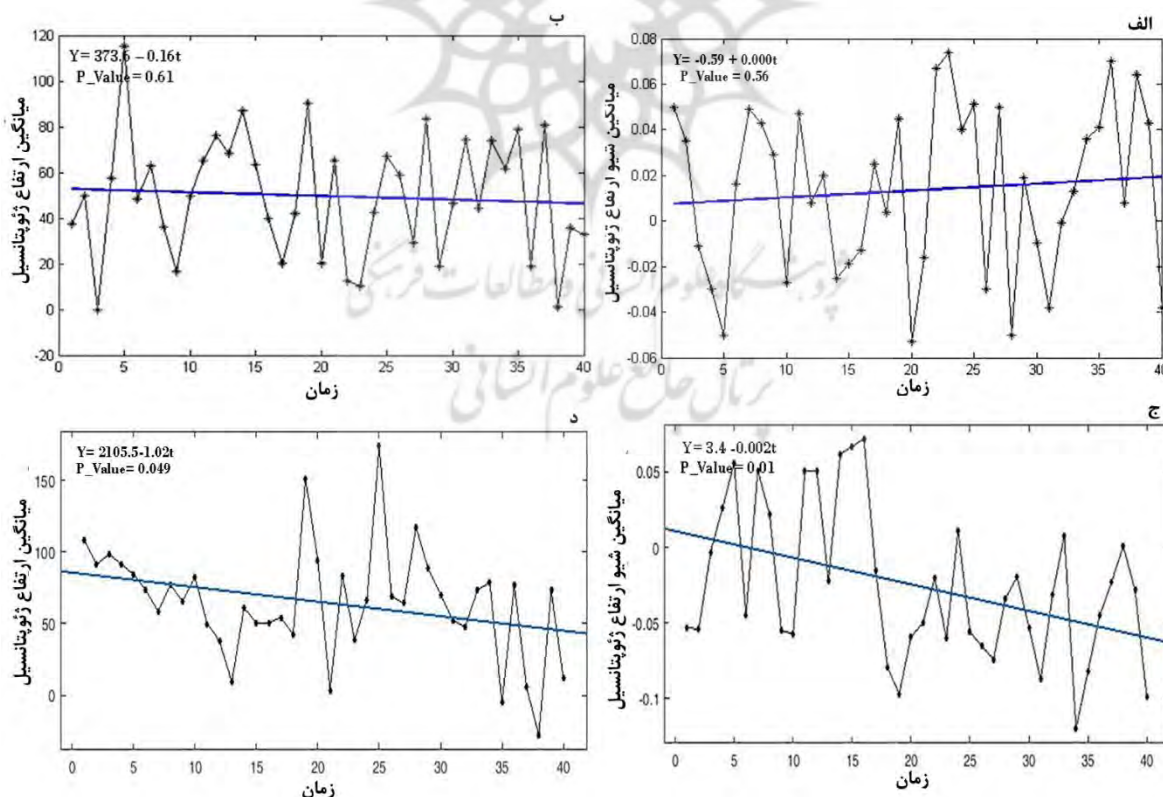
شکل ۵. روند تغییرات سالانه الف) شیو ارتفاع ژئوپتانسیل و ب) ارتفاع ژئوپتانسیل چرخندهای دریای سرخ، ج) شیو ارتفاع ژئوپتانسیل و د) ارتفاع ژئوپتانسیل چرخندهای دریای مدیترانه طی ۱۹۷۹-۲۰۱۸
