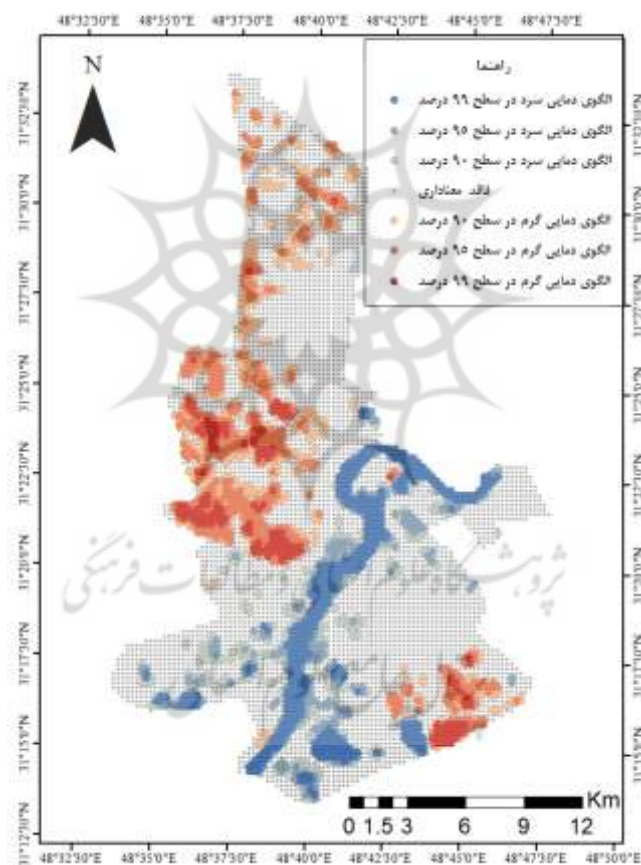
شکل (۵). جزایر حرارتی استخراج شده شهر اهواز مورخه ۲۰۰۱/۰۸/۲۹
