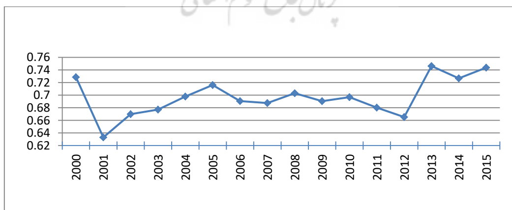
شکل (۳). خروجی خودهمبستگی فضایی موران عمومی (شاخص موران) دمای سطح زمین سال‌های ۲۰۰۰ تا ۲۰۱۵
