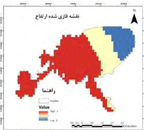
شکل ۴. نقشه فازی ارتفاع
