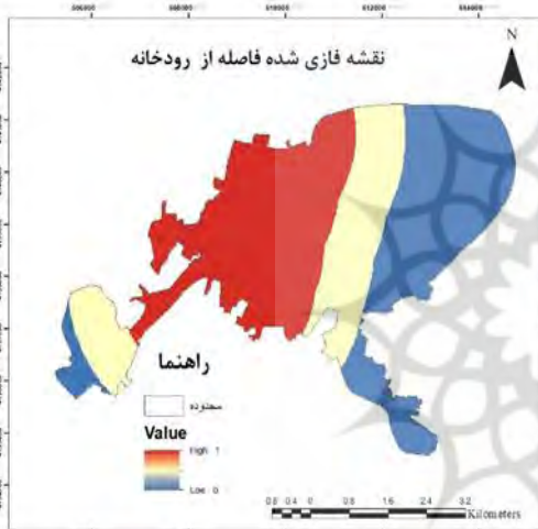
شکل ۷. نقشه فازی فاصله از رودخانه
