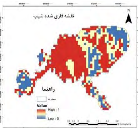
شکل ۵. نقشه فازی شیب
