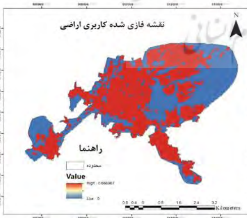
شکل ۹. نقشه فازی کاربری اراضی
