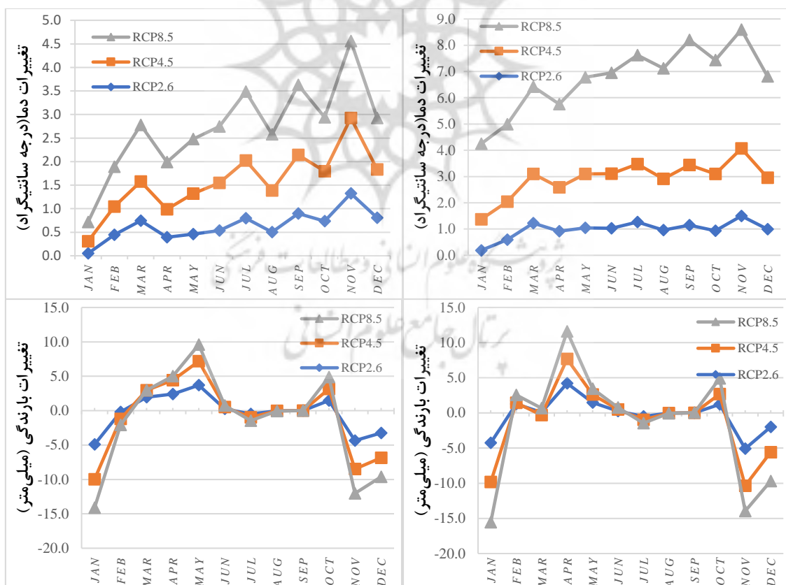
شکل ۱۰. تغییرات ماهانه میانگین دما و مجموع بارندگی پیش‌نگری شده برای دو مدل مورد مطالعه در ایستگاه ندوشن نسبت به دوره پایه تحت سه سناریو وادشت‌تابشی (RCP8.5, 4.5, 2.6) در آینده نزدیک (سمت چپ) و آینده دور (سمت راست)
