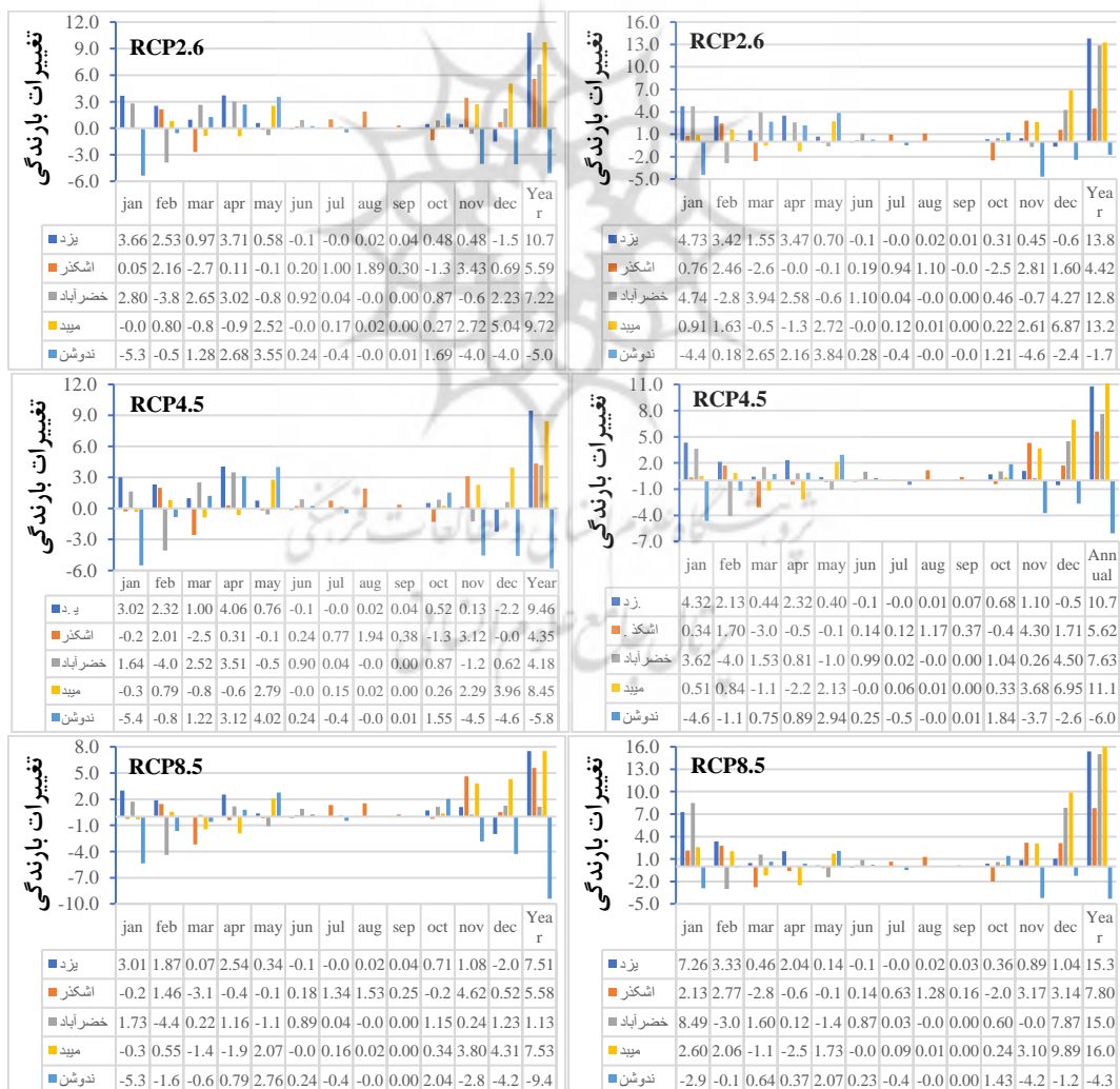
شکل ۶. تغییرات ماهانه بارندگی پیش‌نگری شده تمام ایستگاه‌ها با مدل BCC-CSM1-1 (سمت چپ) و مدل NorESM1-M (سمت راست) نسبت به دوره پایه در سه سناریوی وادشت‌تابشی (RCP2.6, RCP4.5, RCP8.5) در آینده نزدیک
