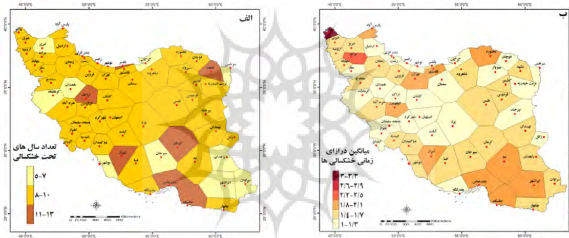
شکل ۵: نقشه‌ی توزیع فضایی الف) تعداد سال‌های تحت خشک‌سالی و ب) میانگین درازای زمانی خشک‌سالی‌های ایران به دست آمده از شاخص بارش استاندارد شده (SPI) برای بازه‌ی زمانی ۱۹۸۶-۲۰۱۵
