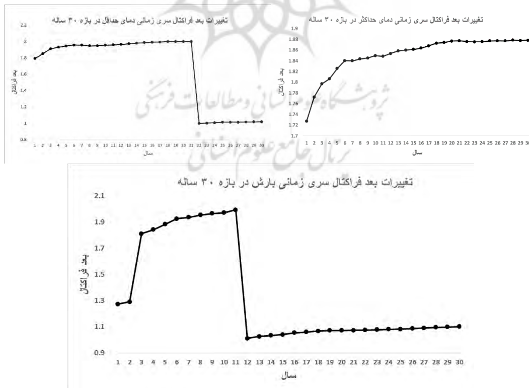
شکل ۳: آنالیز بعد فراکتال سری زمانی دیتاهای ۳۰ ساله‌ی ایستگاه سینوپتیک سد درودزن (۱۹۸۸-۲۰۱۷)
