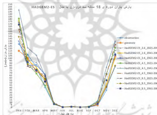
شکل ۱۵: مقایسه میانگین مجموع بارش ماهیانه‌ی مشاهداتی در دوره‌ی ۱۸ ساله سد درودزن (۱۹۹۸-۲۰۰۵) و پیش‌بینی‌شده توسط مدل HadGEM2-ES برای سه دوره‌ی آتی (۲۰۲۱-۲۰۴۰، ۲۰۴۱-۲۰۶۰، ۲۰۶۱-۲۰۸۰) تحت RCP2.6، RCP4.5 و RCP8.5
