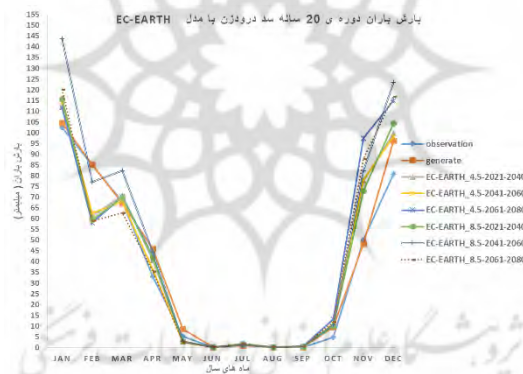
شکل ۹: مقایسه‌ی میانگین مجموع بارش ماهیانه‌ی مشاهداتی در دوره‌ی ۲۰ ساله‌ی سد درودزن (۱۹۹۸-۲۰۱۷) و پیش‌بینی‌شده توسط مدل EC-EARTH برای سه دوره‌ی آتی (۲۰۲۱-۲۰۴۰، ۲۰۴۱-۲۰۶۰، ۲۰۶۱-۲۰۸۰) تحت RCP4.5 و RCP8.5
