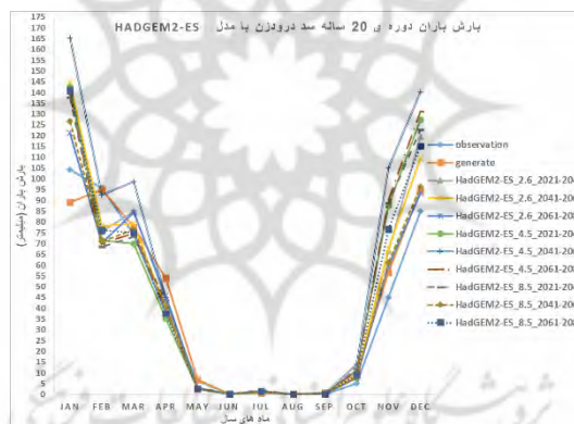
شکل ۱۱: مقایسه‌ی میانگین مجموع بارش ماهیانه‌ی مشاهداتی در دوره‌ی ۲۰ ساله‌ی سد درودزن (۱۹۹۸-۲۰۱۷) و پیش‌بینی‌شده توسط مدل HadGEM2-ES برای سه دوره‌ی آتی (۲۰۲۱-۲۰۴۰، ۲۰۴۱-۲۰۶۰، ۲۰۸۰-۲۰۶۱) تحت RCP2.6، RCP4.5 و RCP8.5
