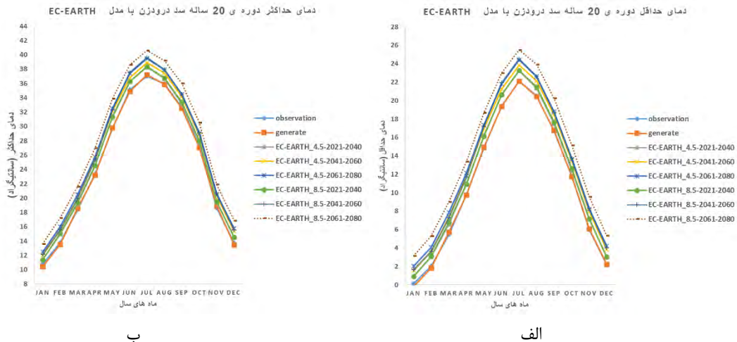
شکل ۸: الف و ب: به ترتیب مقایسه‌ی میانگین ماهیانه‌ی دمای حداقل و حداکثر مشاهداتی در دوره‌ی ۲۰ ساله‌ی سد درودزن (۱۹۹۸-۲۰۱۷) و پیش‌بینی‌شده توسط مدل EC-EARTH برای سه دوره‌ی آتی (۲۰۲۱-۲۰۴۰، ۲۰۴۱-۲۰۶۰، ۲۰۶۱-۲۰۸۰) تحت RCP4.5 و RCP8.5 (۲۰۶۱)
